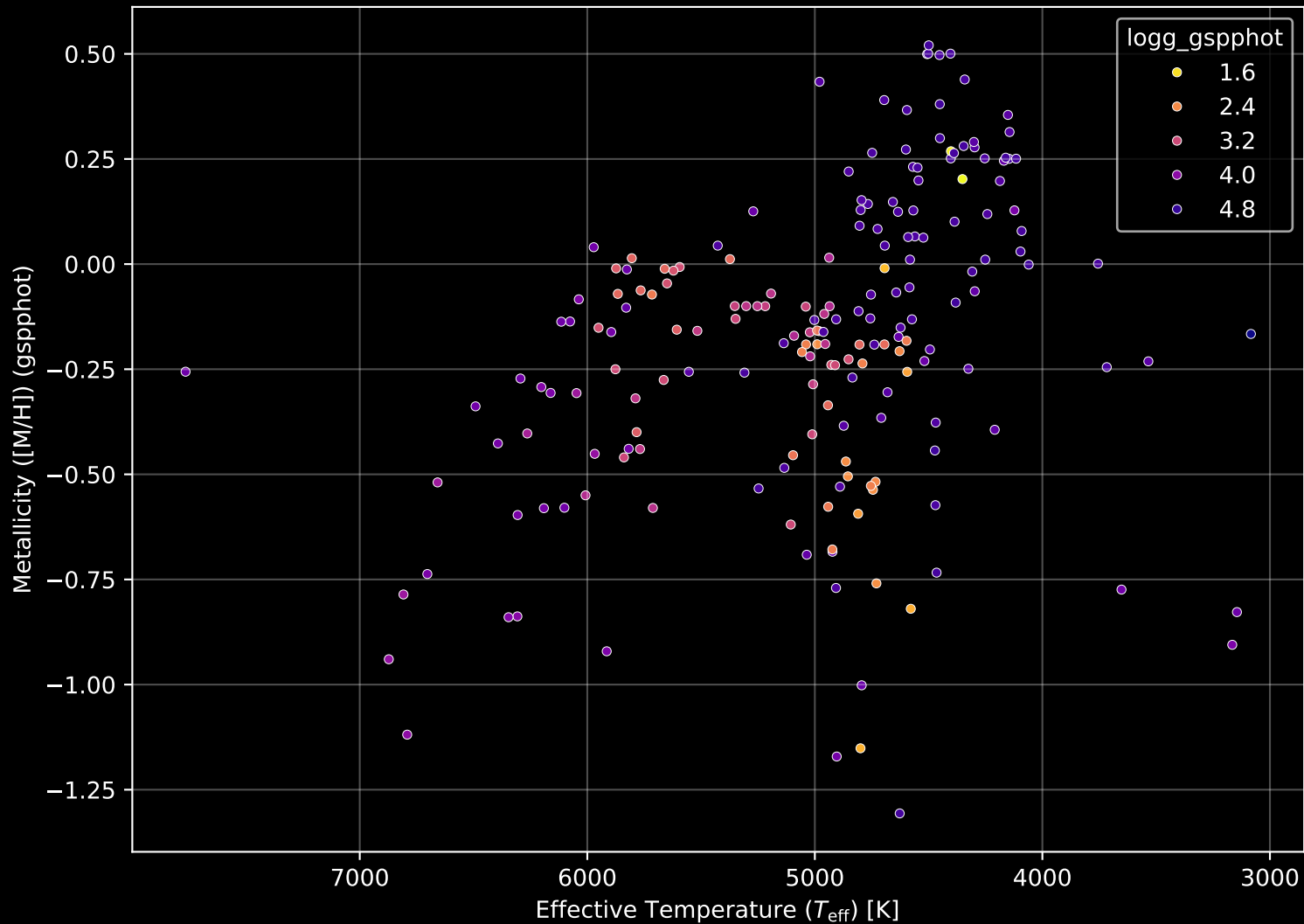
APOGEE DR17 Field: [325+76] Stellar Population Parameters (n= 194)
